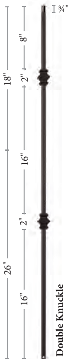
Double Knuckle 9007TB- * -44 10 pcs per box 420 pcs per skid
